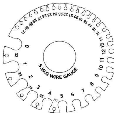
Fig: Wire Gauge
